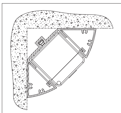
> Medienkanal für Eckmontage aus Aluminium, Artikelnr. 650 100
